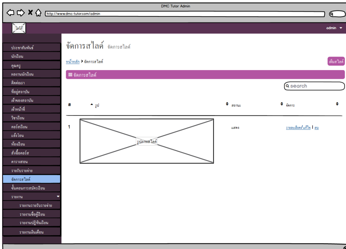
ภาพที่ 3.56 หน้าจอสำหรับจัดการสไลด์หน้าเว็บไซต์
