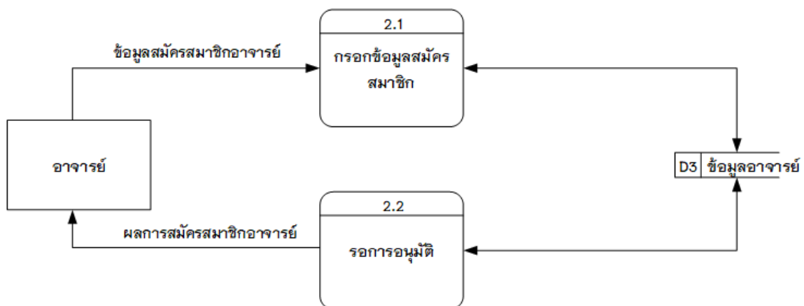
ภาพที่ 3.7 แผนภาพกระแสข้อมูล DFD Level 1 โปรเซสที่ 2 สมัครสมาชิกอาจารย์
