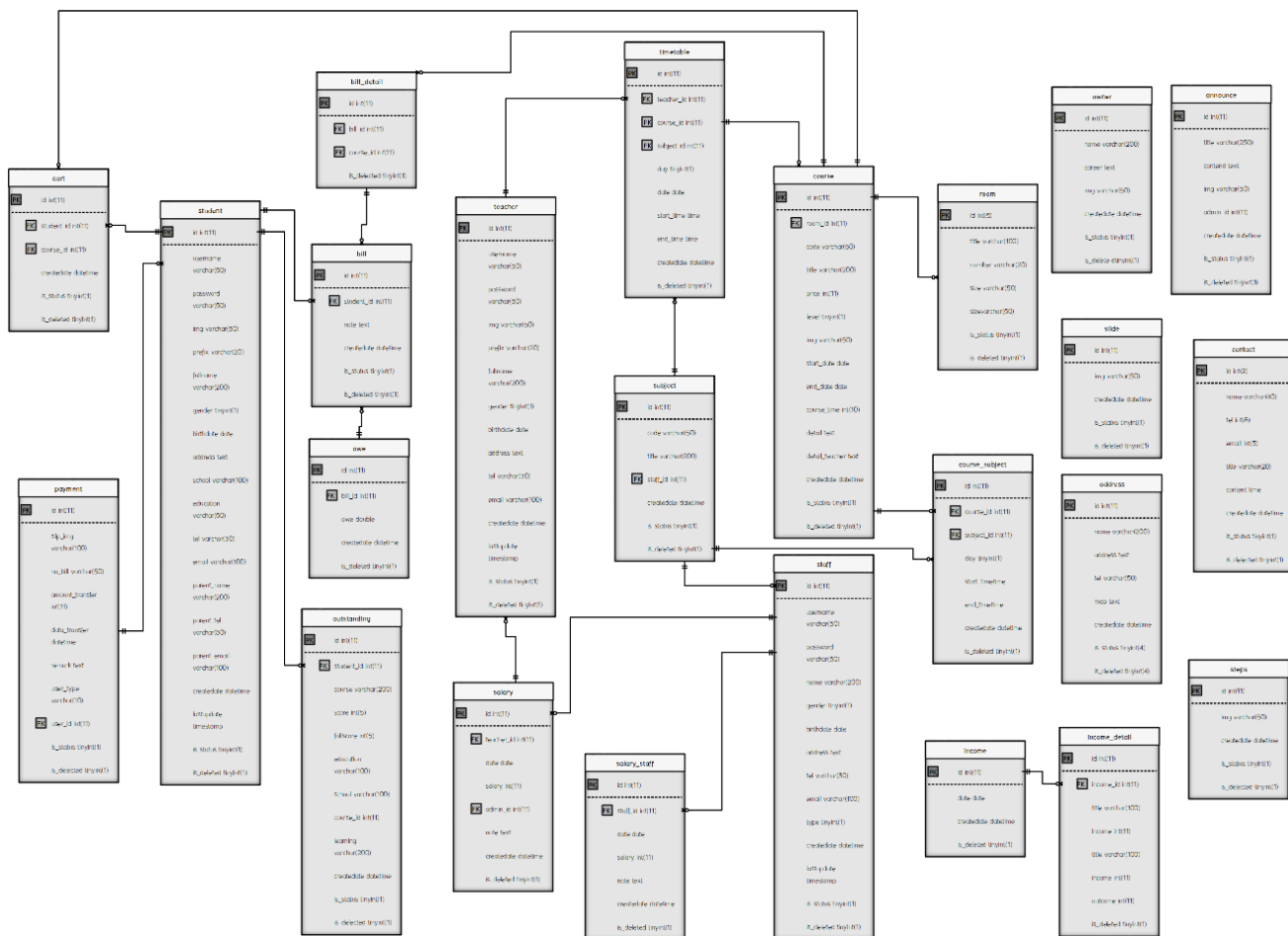
ภาพที่ 3.9 แผนภาพความสัมพันธ์ของฐานข้อมูลแบบ Crow's Foot Model
