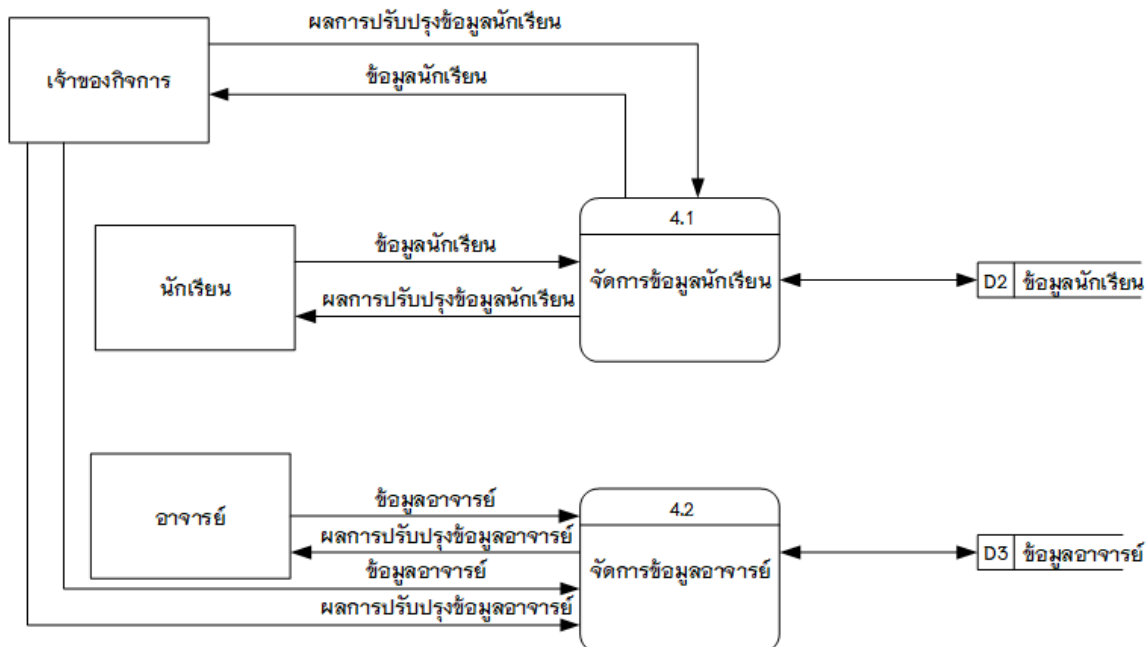
ภาพที่ 3.8 แผนภาพกระแสข้อมูล DFD Level 1 โปรเซสที่ 4 จัดการข้อมูลผู้ใช้
