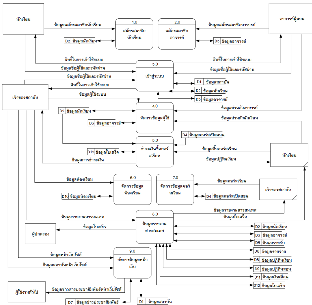
ภาพที่ 3.5 แผนภาพกระแสข้อมูล DFD Level 0 ระบบการพัฒนาระบบ บริหาร จัดการสถาบันกวดวิชา DMC ลำปาง
