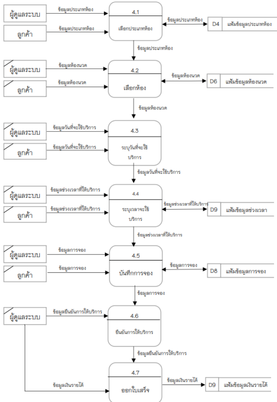
ภาพที่ 3.8 แสดงแผนภาพ Data Flow Diagram Level 1 Process 4 .0
