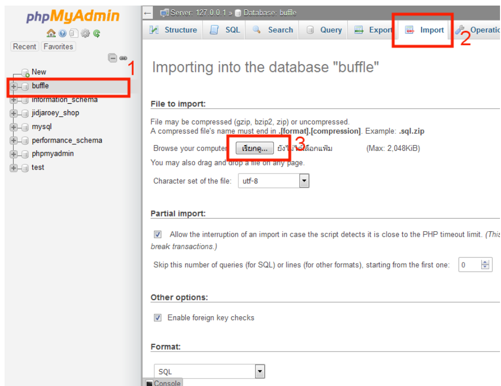
ภาพที่ ก.2.5 หน้าแสดงขั้นตอนการเพิ่มฐานข้อมูล ขั้นตอนที่ 3
