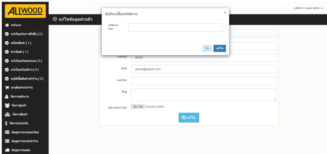
ภาพที่ 4.6 ภาพแสดงหน้าจอภาพสำหรับตั้งรหัสผ่านใหม่
