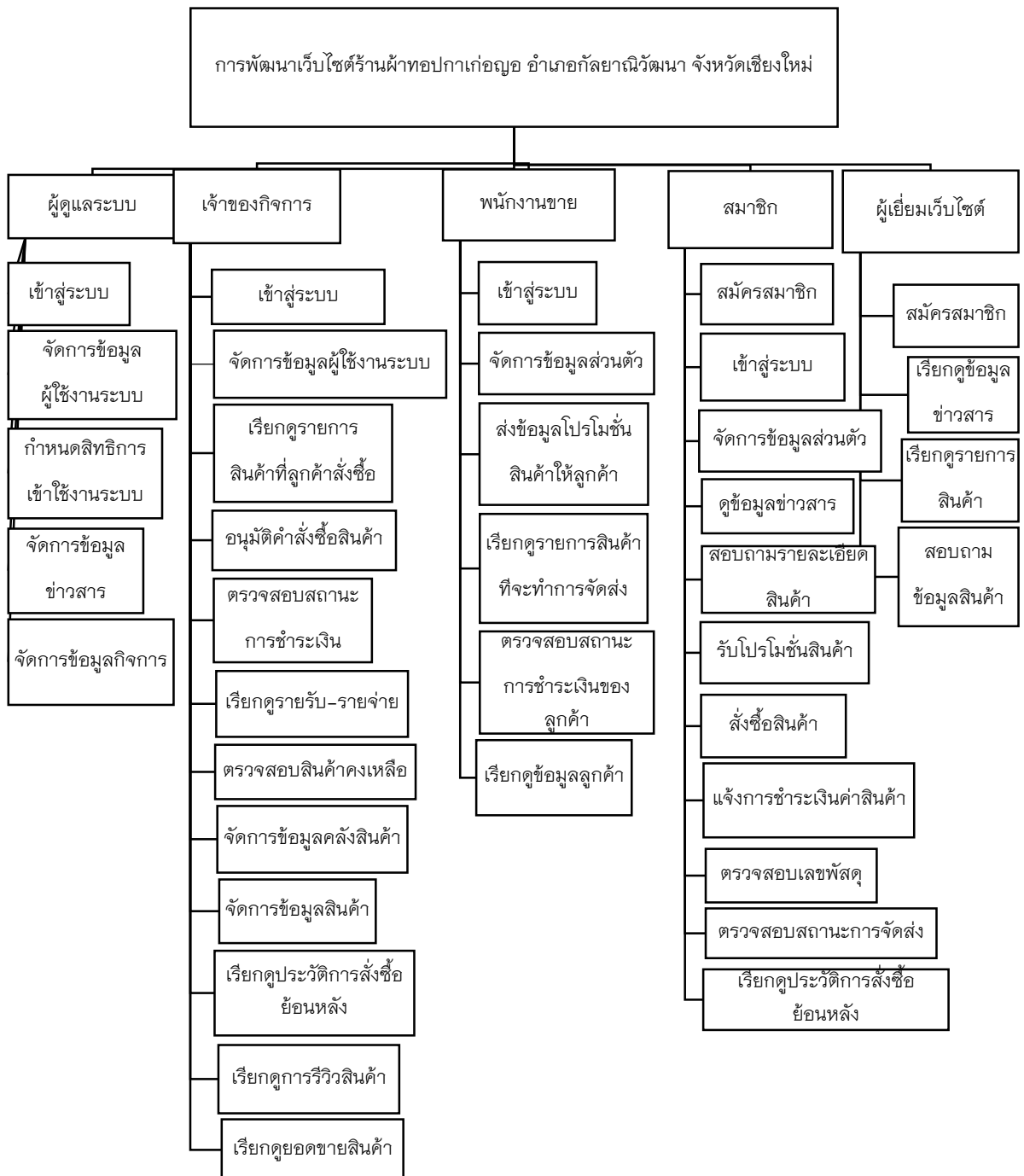
ภาพที่ 3.10 แผนภาพโครงสร้างระบบ
