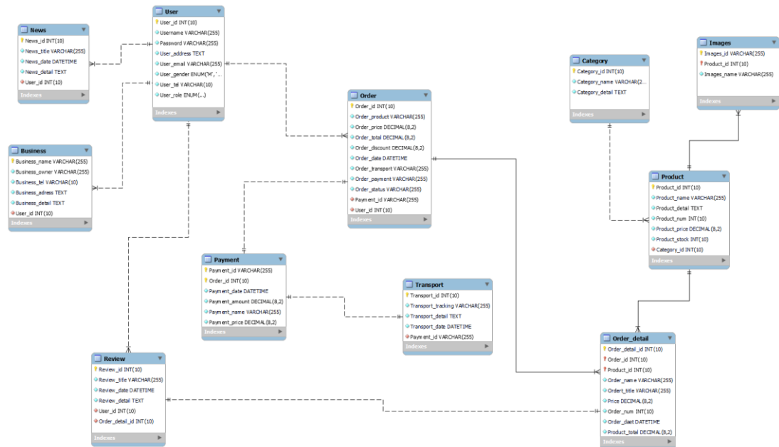
ภาพที่ 3.9 ความสัมพันธ์ของฐานข้อมูลแบบ Crow's Foot Mod
