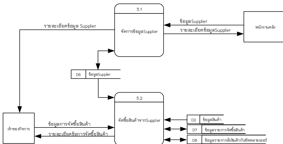
ภาพที่ 3.8 แผนภาพกระแสข้อมูลระดับที่ 1 กระบวนการที่ 3
