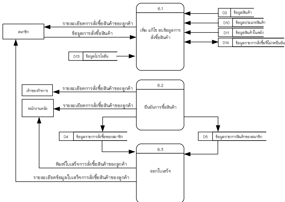
ภาพที่ 3.10 แผนภาพกระแสข้อมูลระดับที่ 1 กระบวนการที่ 6
