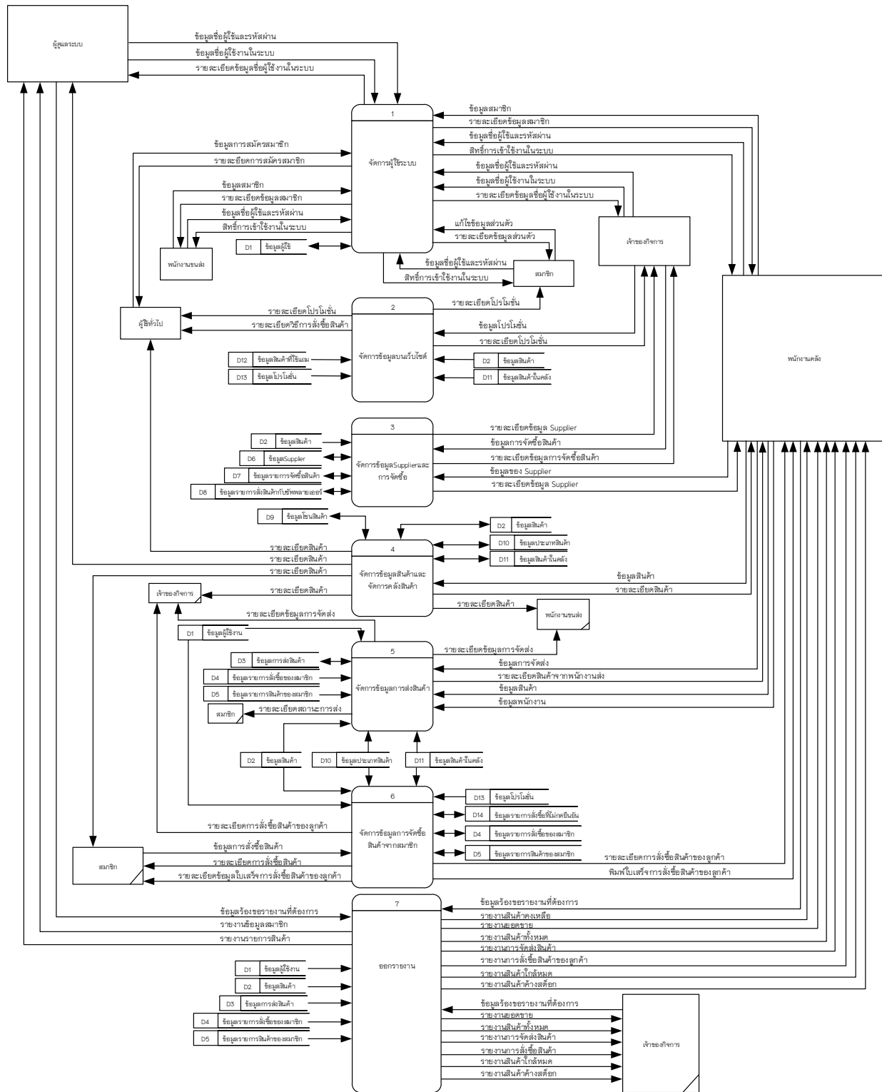
ภาพที่ 3.6 แผนภาพกระแสข้อมูล (Data Flow Diagram Level 0)
