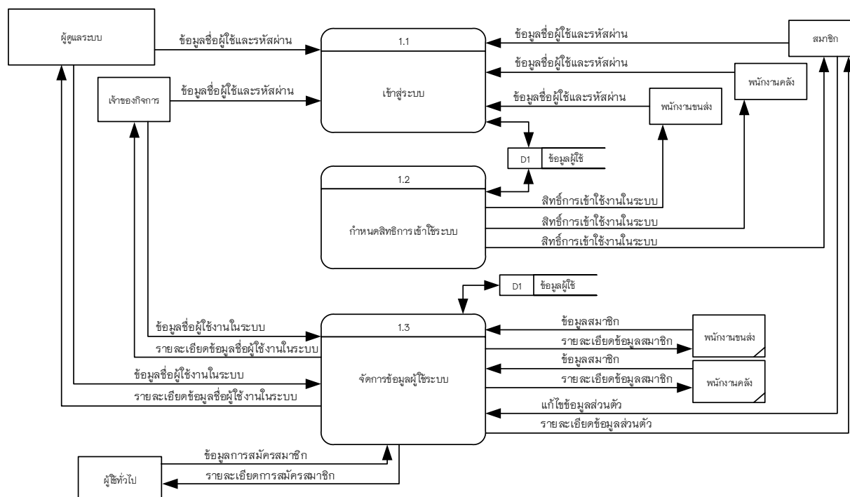
ภาพที่ 3.7 แผนภาพกระแสข้อมูลระดับที่ 1 กระบวนการที่ 1
