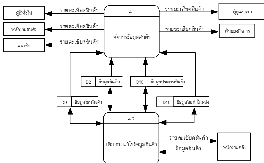
ภาพที่ 3.9 แผนภาพกระแสข้อมูลระดับที่ 1 กระบวนการที่ 4
