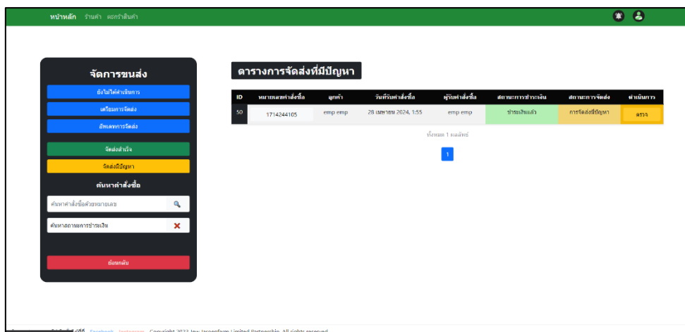
ภาพที่ 4.54 หน้าจอแสดงสถานะการจัดส่งที่มีปัญหา
