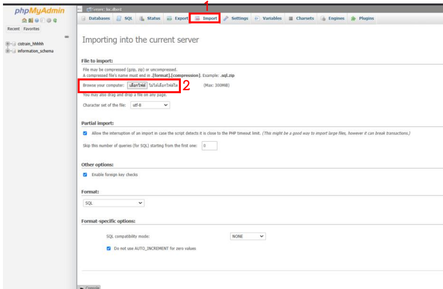
ภาพที่ ก.6 หน้าจอ Import ไฟล์ฐานข้อมูล
