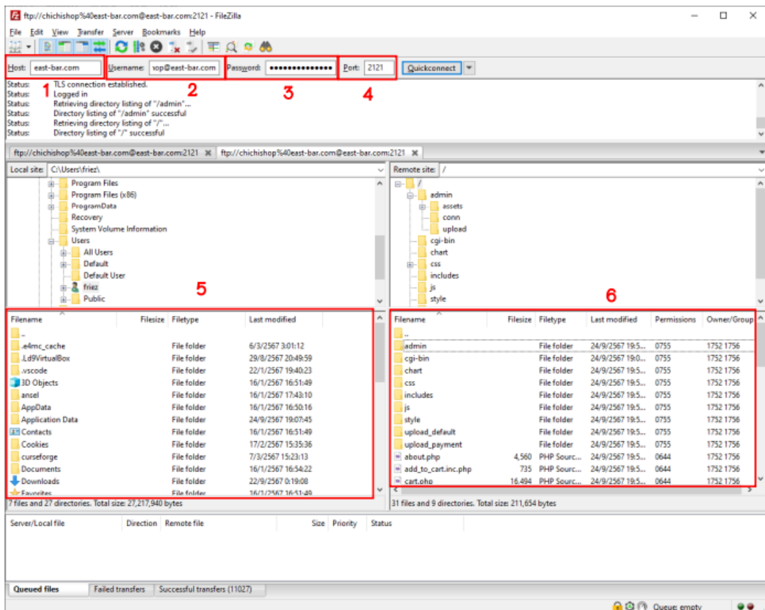
ภาพที่ ก.1 หน้าจอโปรแกรมไฟล์ซิลลาลงข้อมูลชื่อและรหัส
