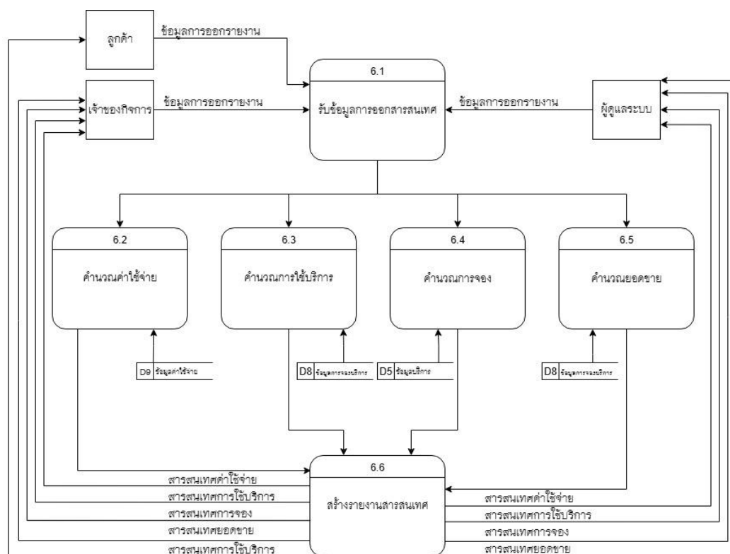
ภาพที่ 3.8 แสดง Data Flow Diagram (DFD) Level 1 Process 6.0 สร้างรายงานสารสนเทศ
