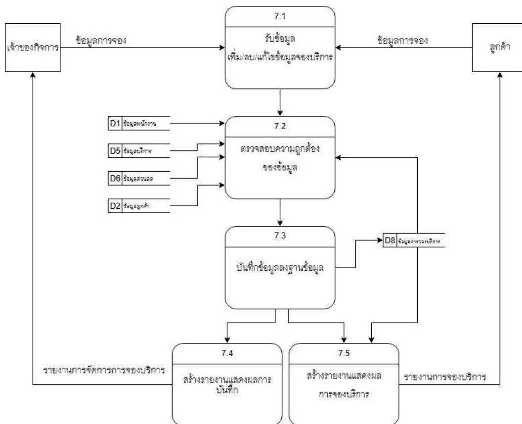
ภาพที่ 3.9 แสดง Data Flow Diagram (DFD) Level 1 Process 7.0 การจองบริการ
