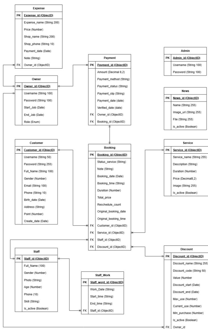
ภาพที่ 3.10 ความสัมพันธ์ของฐานข้อมูล Crow's Foot Mode
