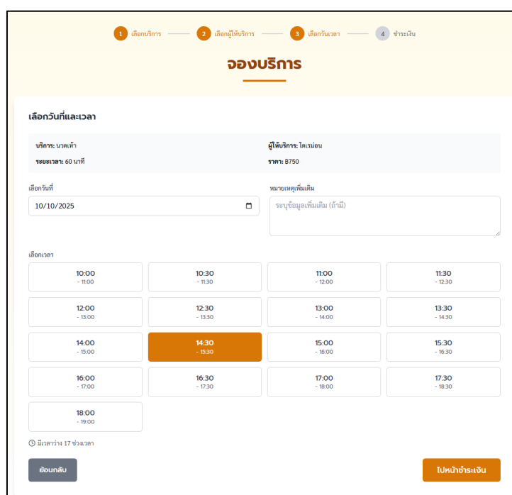
ภาพที่ 4.22 หน้าจอสำหรับเลือกวันที่และช่วงเวลาที่ต้องการ จากภาพที่ 4.22 หน้าจอแสดงการเลือกวันที่และช่วงเวลา เป็นขั้นตอนที่สามของการจอง โดย จะต้องเลือกวันที่ก่อน ระบบถึงจะแสดงช่วงเวลาที่มีพนักงานว่าง
