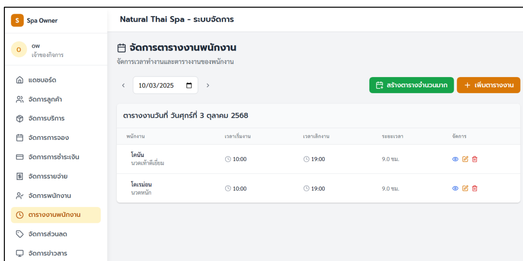
ภาพที่ 4.8 หน้าแสดงระบบจัดการตารางงานพนักงาน
