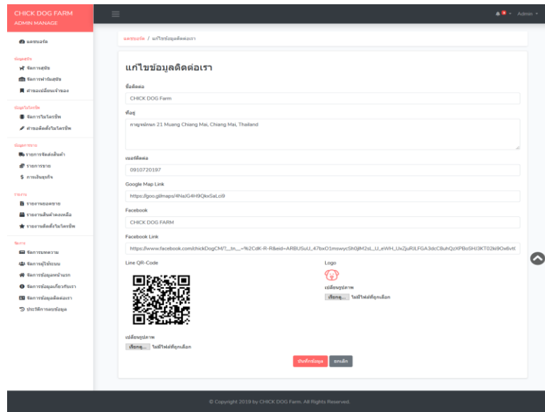
ภาพที่ 4.54 แสดงหน้าจัดการข้อมูลติดต่อเรา
