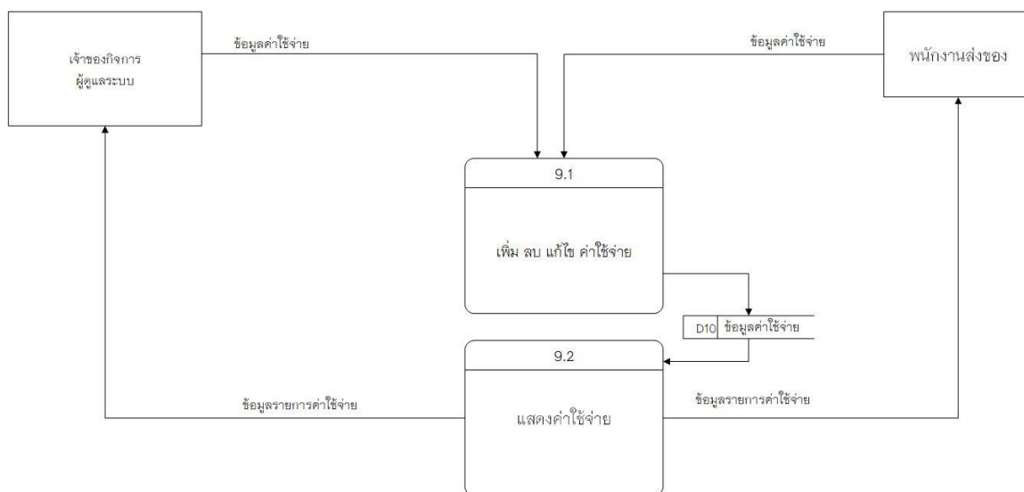
ภาพที่ 3.13 แผนภาพกระแสข้อมูลระดับที่ 1 (Data Flow Diagram Level 1 Process 9.0)
