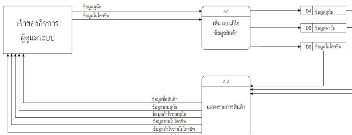
ภาพที่ 3.9 แผนภาพกระแสข้อมูลระดับที่ 1 (Data Flow Diagram Level 1 Process 3.0)
