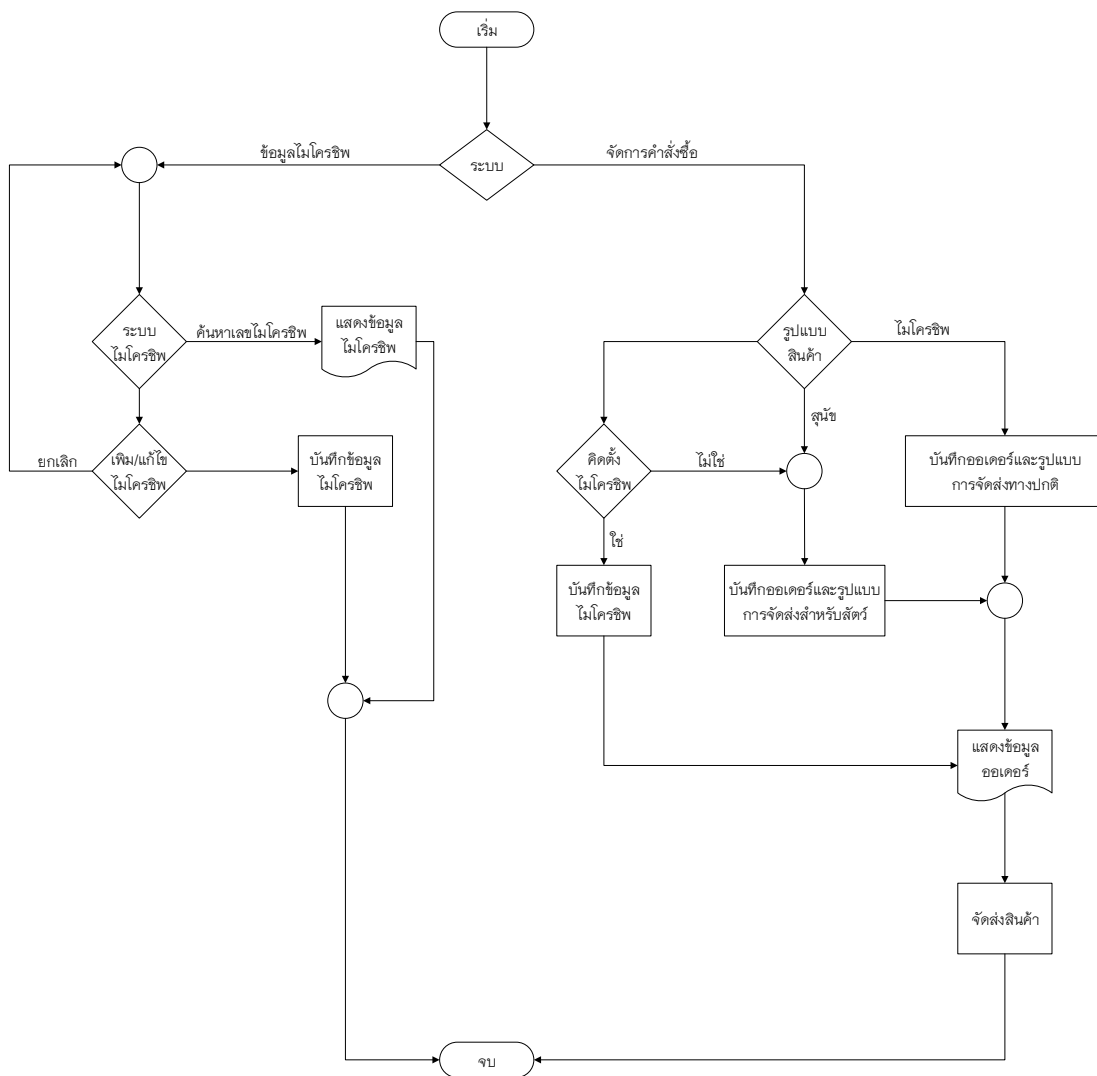
ภาพที่ 3.4 แสดงแผนผังการทำงานในระบบงานใหม่
