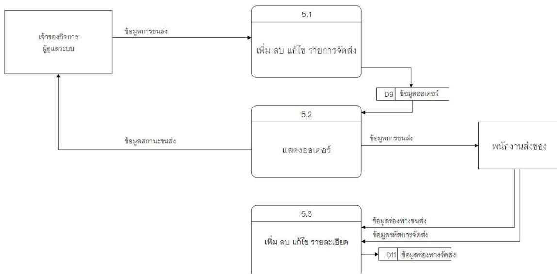
ภาพที่ 3.10 แผนภาพกระแสข้อมูลระดับที่ 1 (Data Flow Diagram Level 1 Process 5.0)
