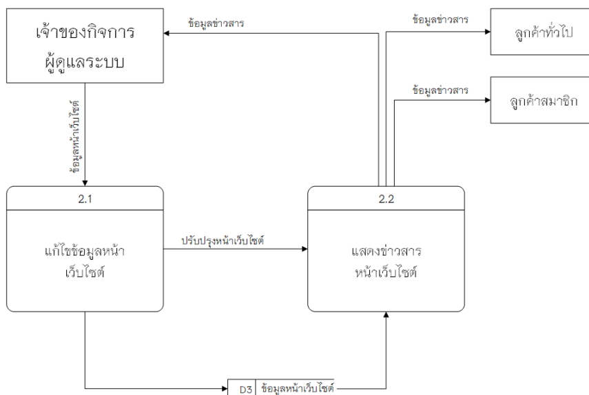
ภาพที่ 3.8 แผนภาพกระแสข้อมูลระดับที่ 1 (Data Flow Diagram Level 1 Process 2.0)
