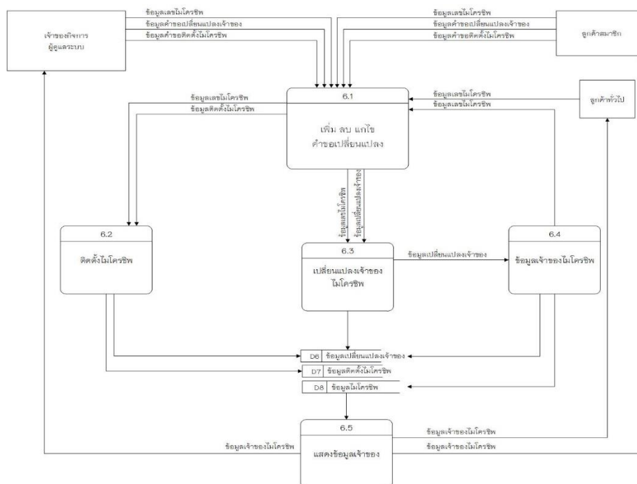
ภาพที่ 3.11 แผนภาพกระแสข้อมูลระดับที่ 1 (Data Flow Diagram Level 1 Process 6.0)
