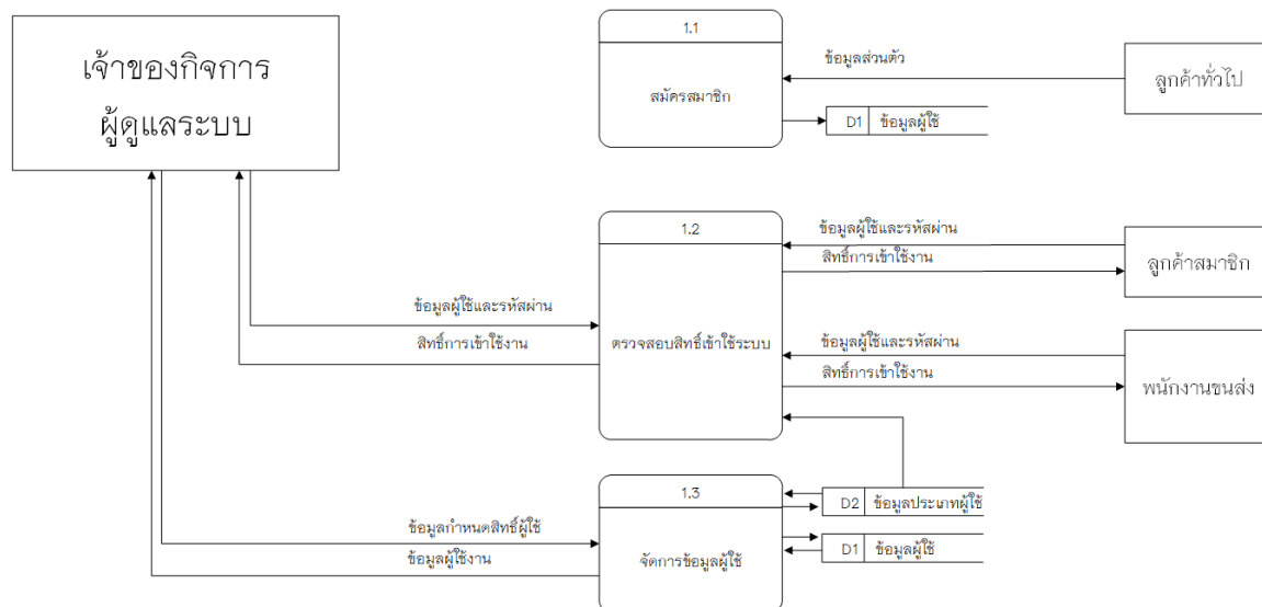
ภาพที่ 3.7 แผนภาพกระแสข้อมูลระดับที่ 1 (Data Flow Diagram Level 1 Process 1.0)
