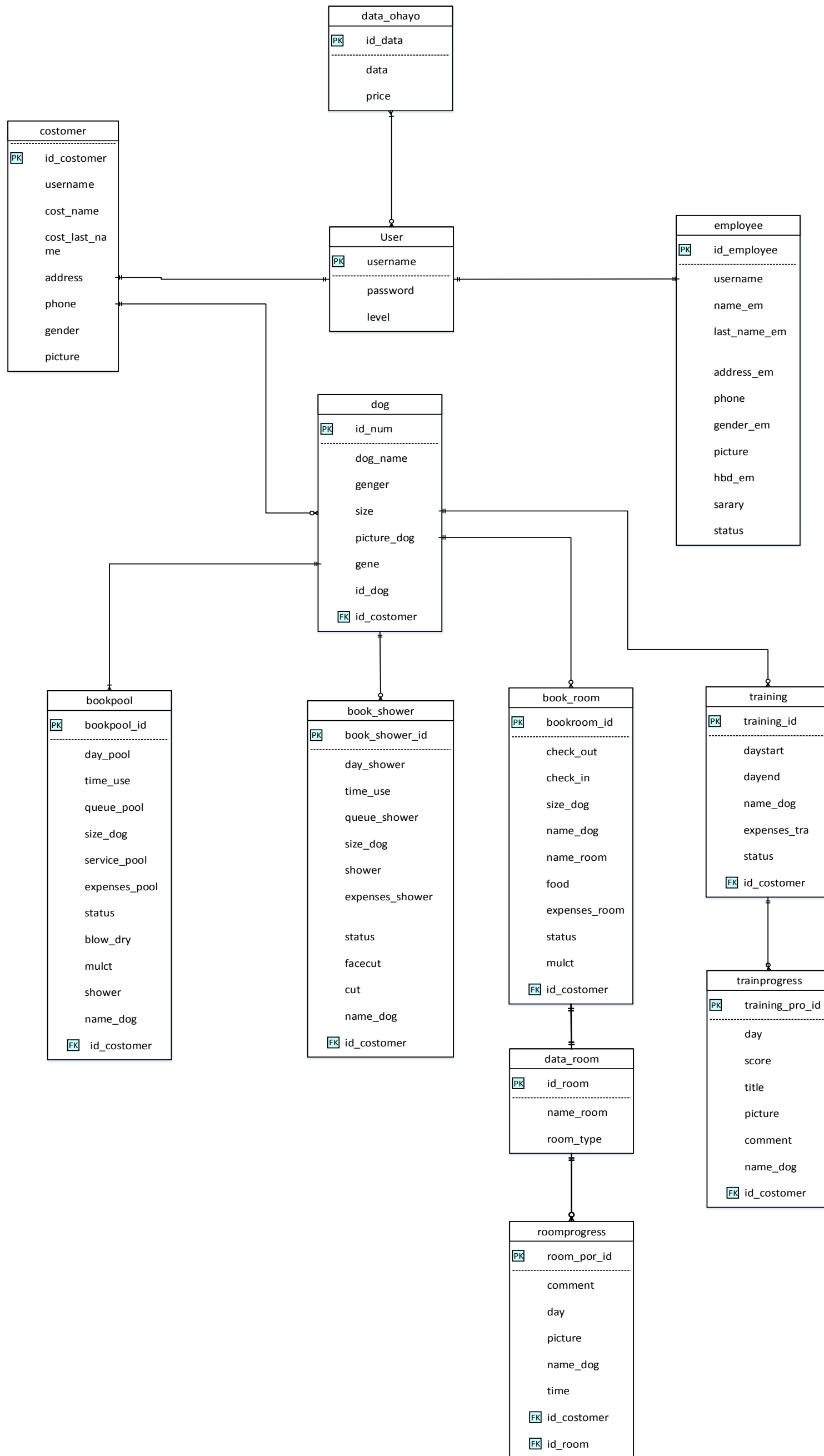
ภาพที่ 3.5 ER-Diagram
