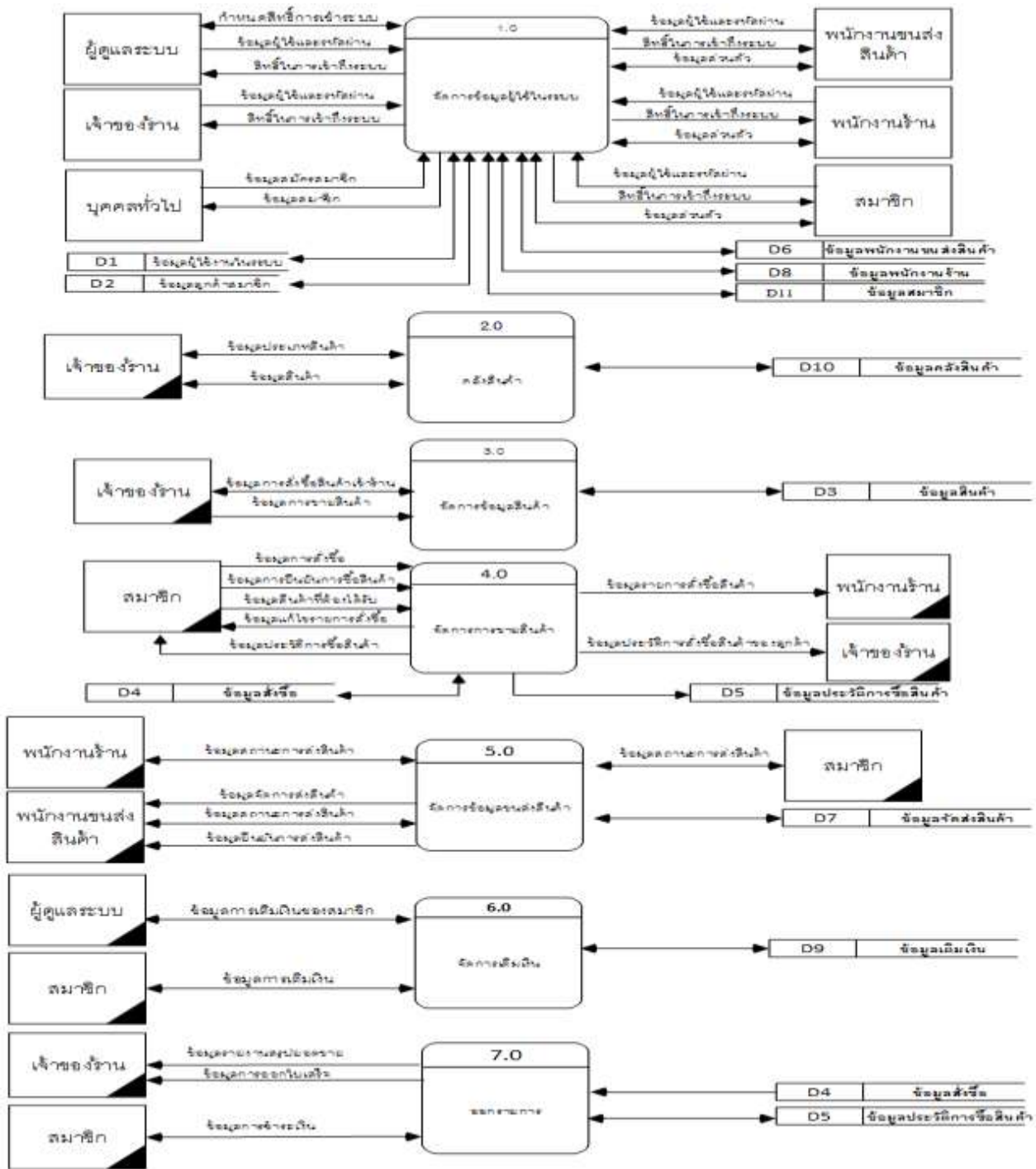
ภาพที่ 3.5 แผนภาพกระแสข้อมูล DFD Level 0 ระบบสารสนเทศการบริหารจัดการร้านค้าปลีกพาณิชย์
